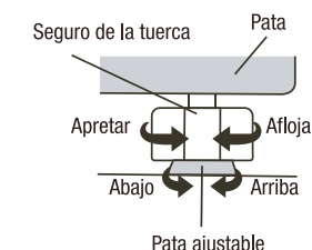
Piso inclinado
